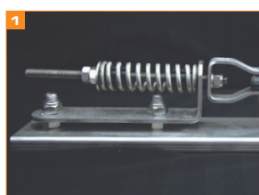
Endschloss: (mit Feder- vorspannung, vormont.)
