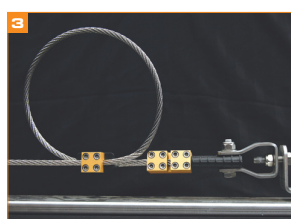
Schockabsorber: (Seilschleife vormontiert)
